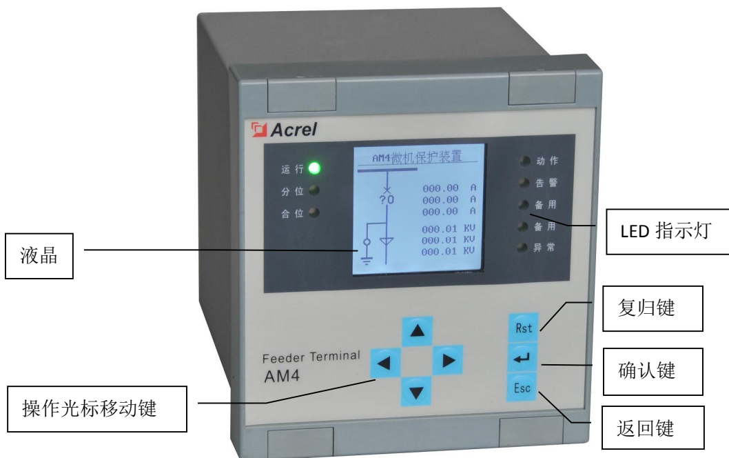
图 3.1 AM4 前面板
