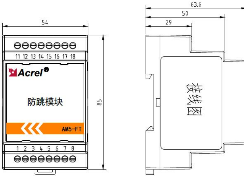
图 C.3 AM5-FT 尺寸图
